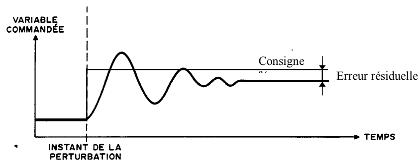
Figure 6-14 L'erreur résiduelle
