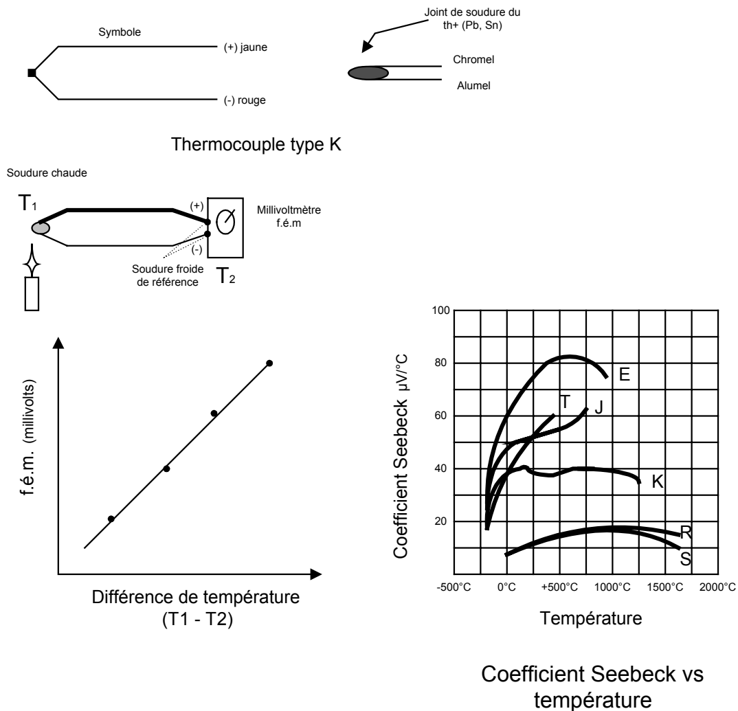
Figure 5-66 : Le thermocouple: symboles et principes
