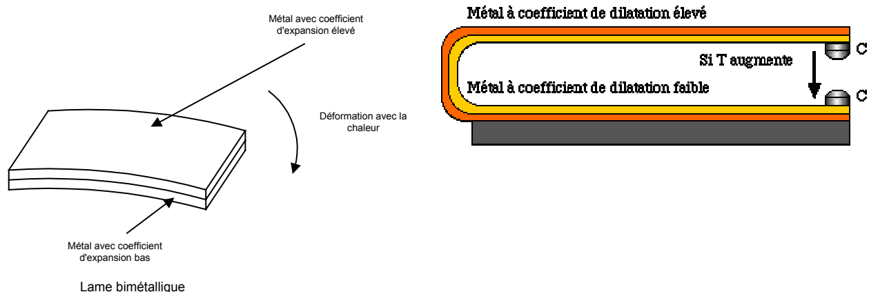
Figure 5-57 : Circuit de commande avec lame bimétallique
