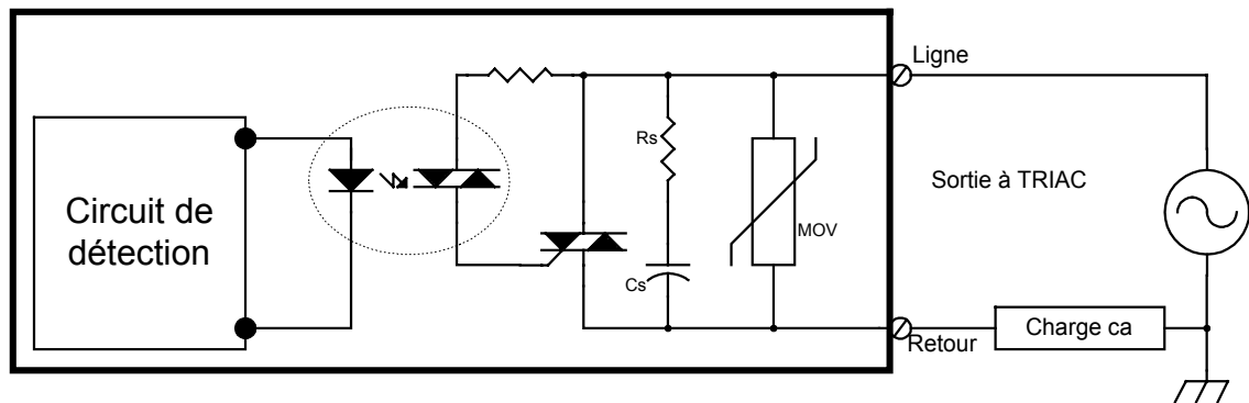
Module de sortie à TRIAC pour charge ca
