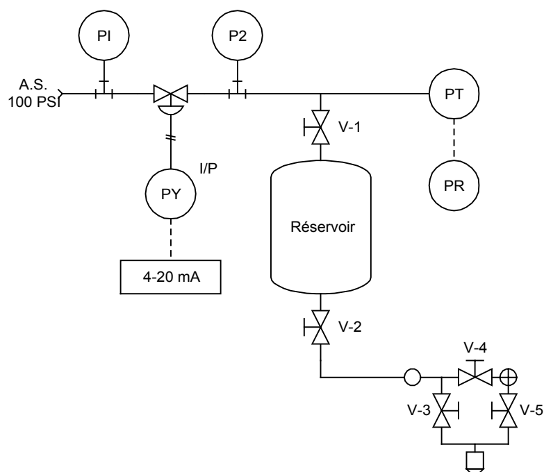
Figure 2-8 Schéma de principe d'un procédé de pression
