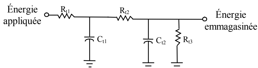
Figure 6-3 Équivalent électrique amélioré de l'échangeur de chaleur
