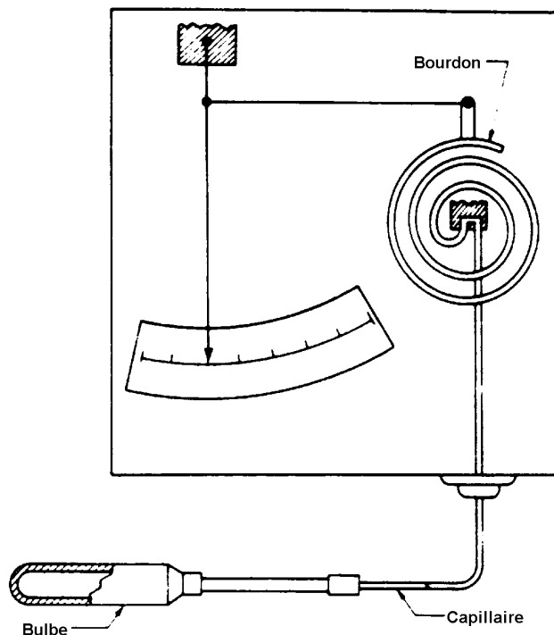
Figure 5-58 : Thermomètre à bulbe
