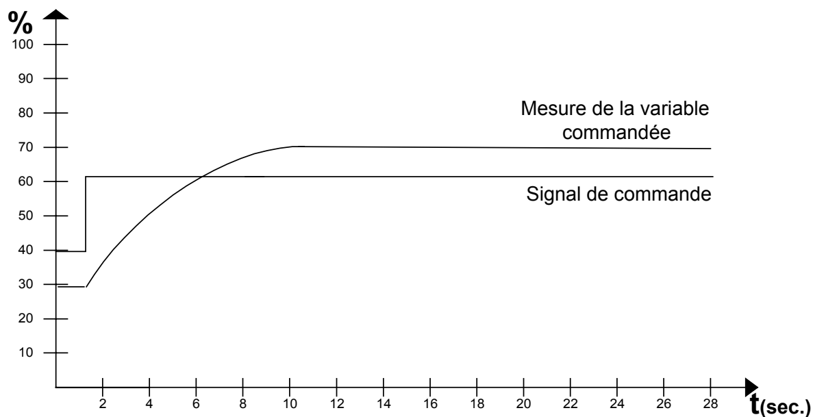
Figure 0-2 Réponse à l'échelon
