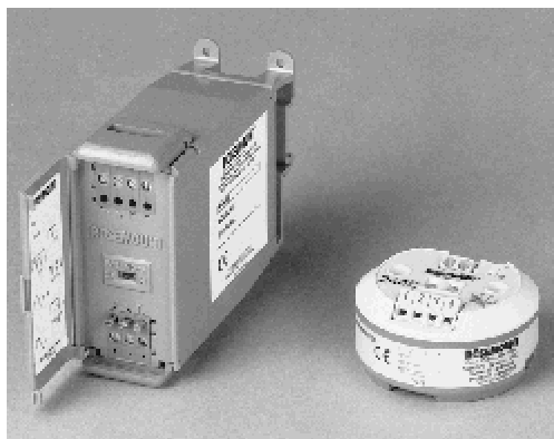
Figure 3-2 Transmetteurs
