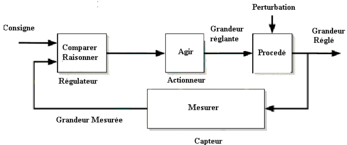
Figure 1-4. Schémas de principe de la régulation
