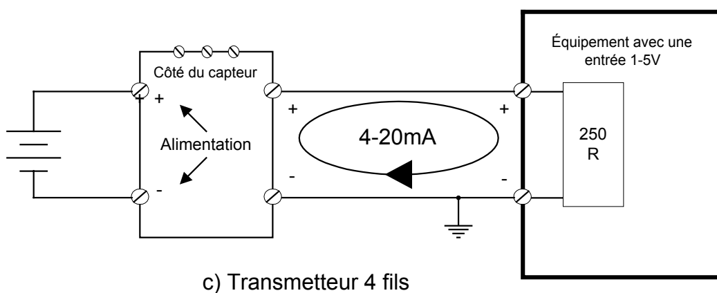
Figure 0-10 : Raccordement d'un transmetteur 4-20mA
