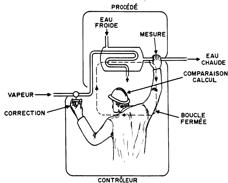
Figure 0-1 L'opérateur joue le rôle de contrôleur dans cette commande de température
