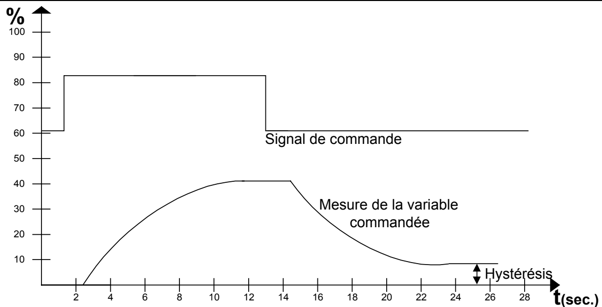
Figure 6-21 Réponse d'un procédé avec hystérésis
