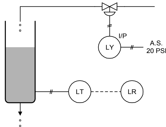
Figure 2-7 Schéma de principe d'un procédé de niveau
