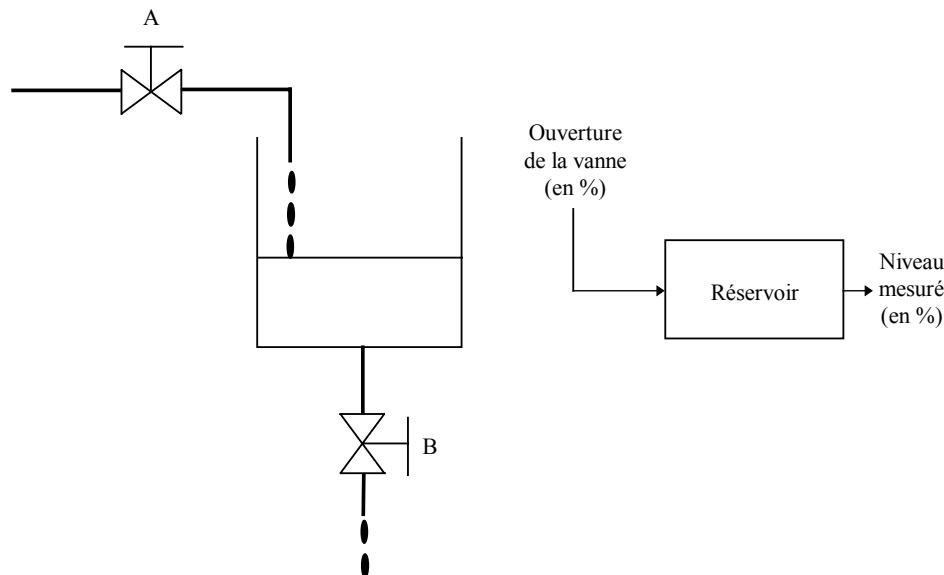
Figure 6-15 Réservoir simple
