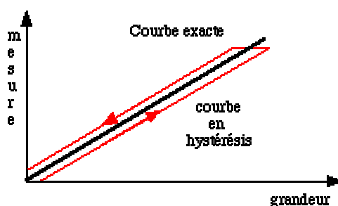
Figure 3-9 Hystérésis
